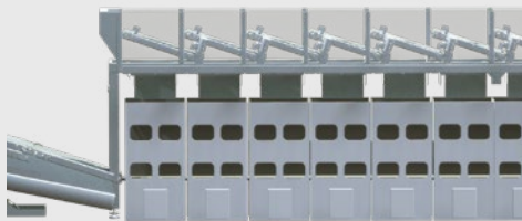
称重料仓 + 料袋轨道系统
