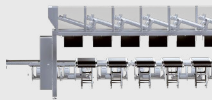
称重输送带 + 料袋轨道系统
